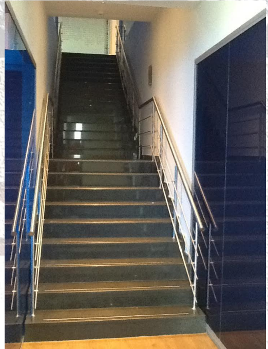
ESCALERA DE GENERAL ELECTRIC: CON VIGA CENTRAL, RECTA, PASOS Y CONTRAPASOS EN GRANITO DE PIEDRA. BARANDA EN ACERO INOXIDABLE
